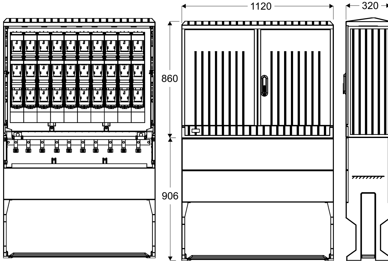
Widok złącza
