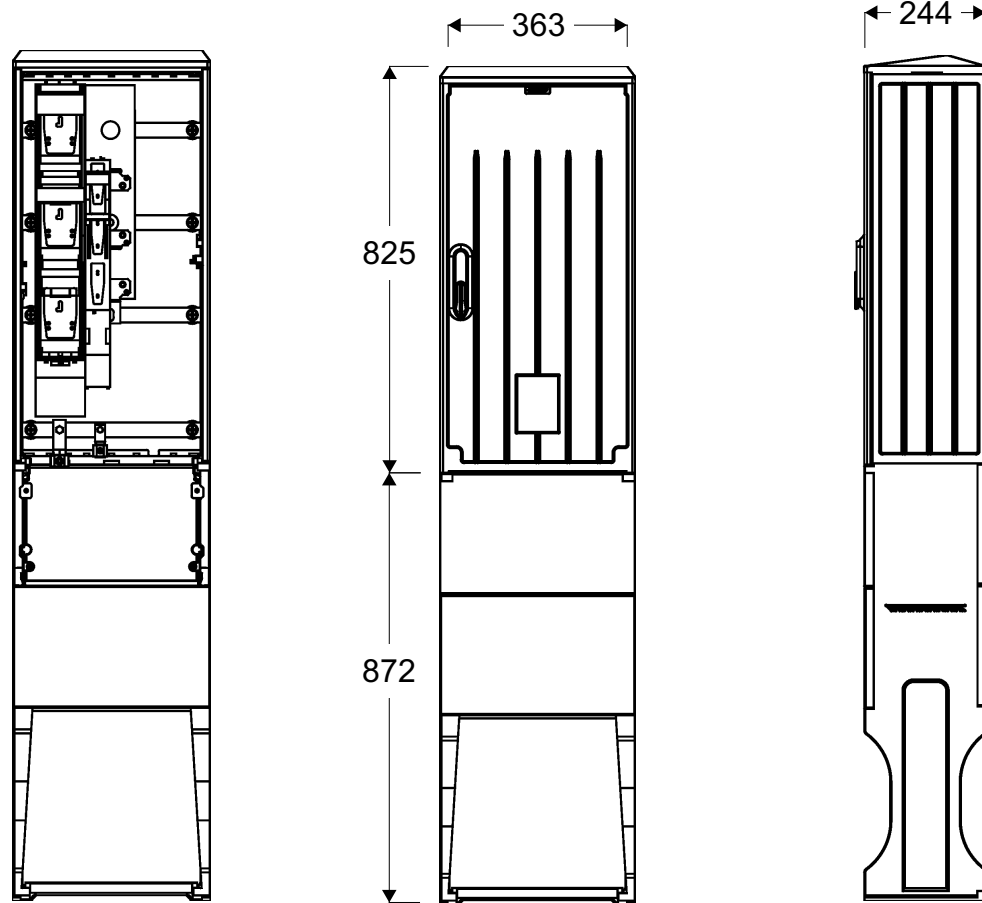
Widok złącza
