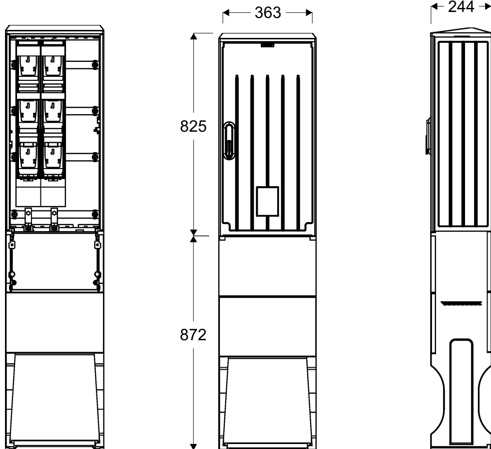
Widok złącza
