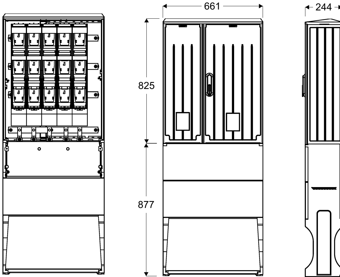
Widok złącza
