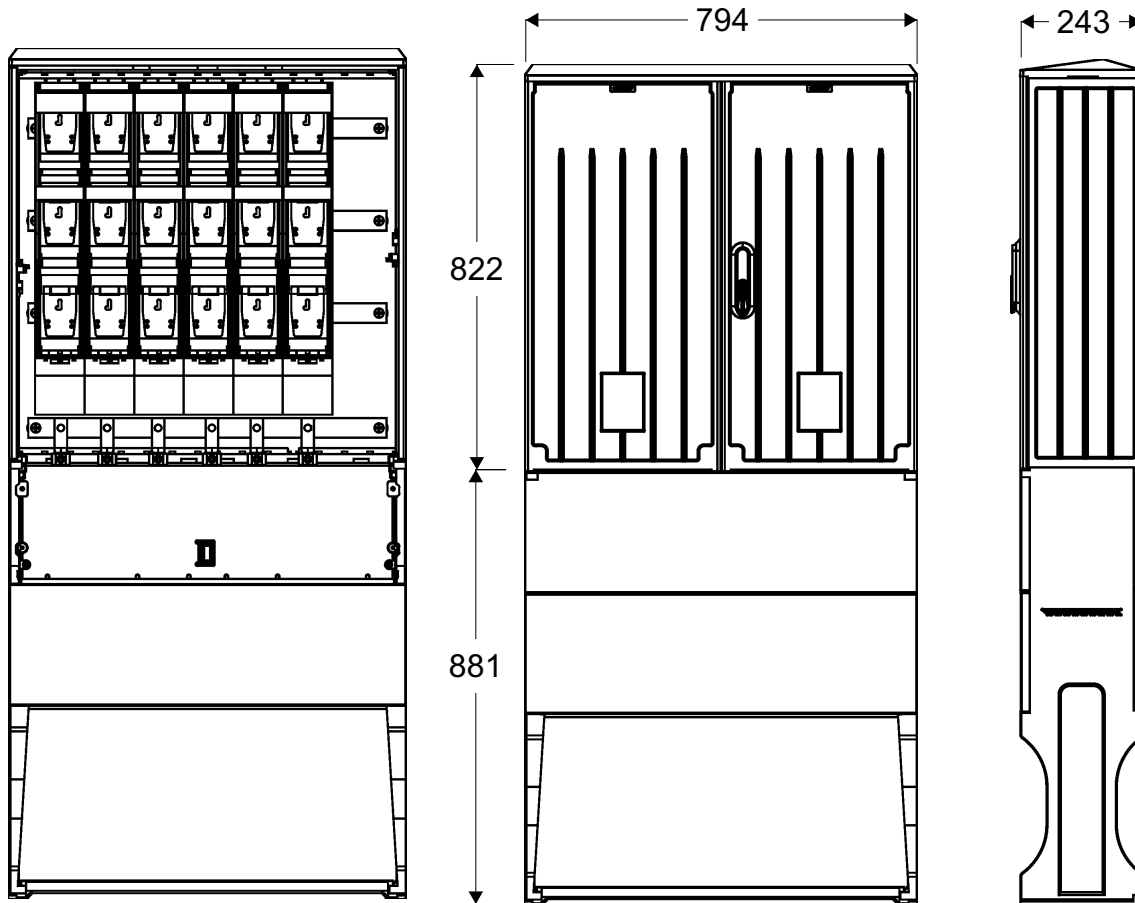
Widok złącza
