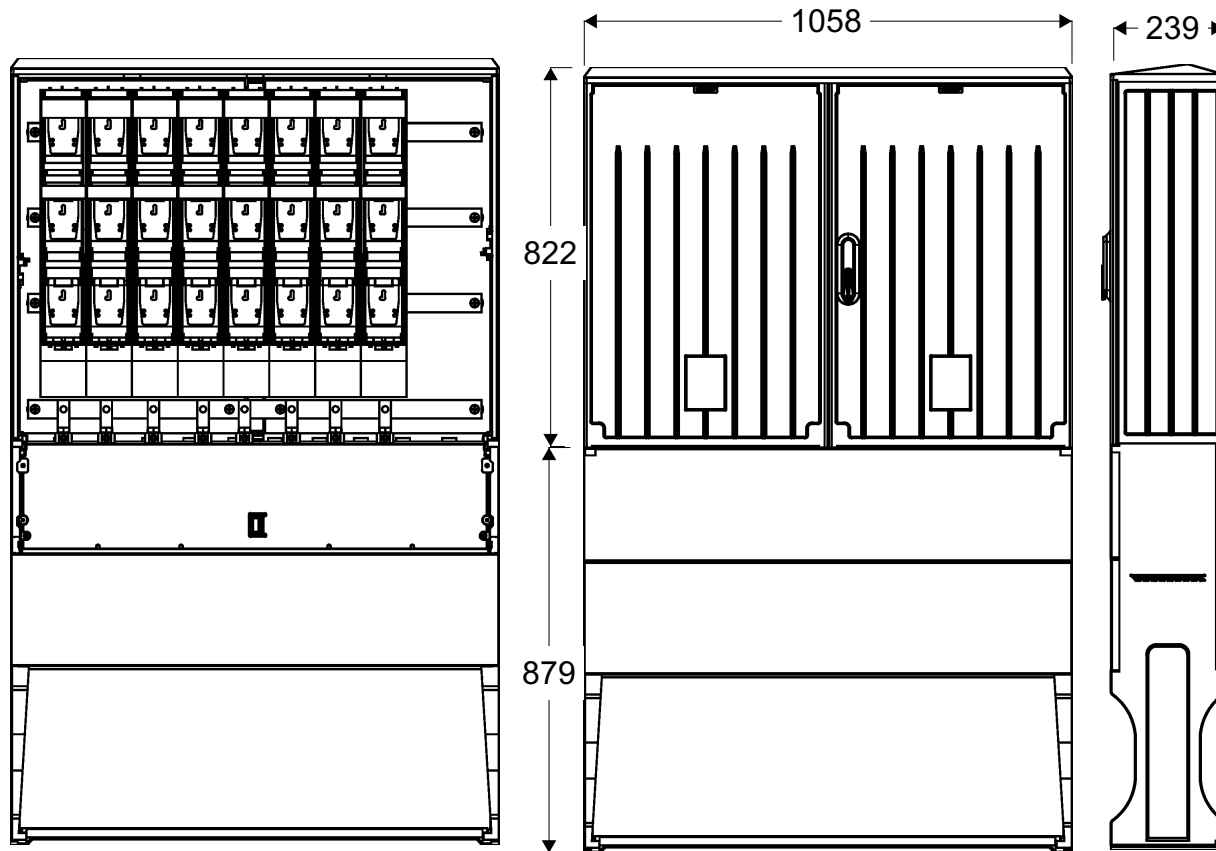
Widok złącza
