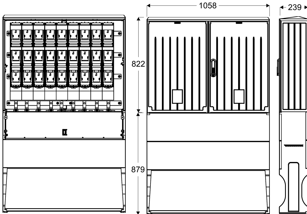
Widok złącza
