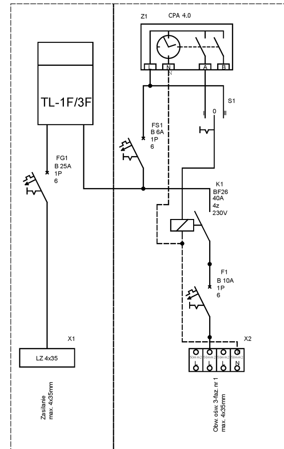
Schemat elektryczny
