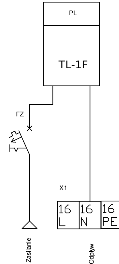
Schemat elektryczny
