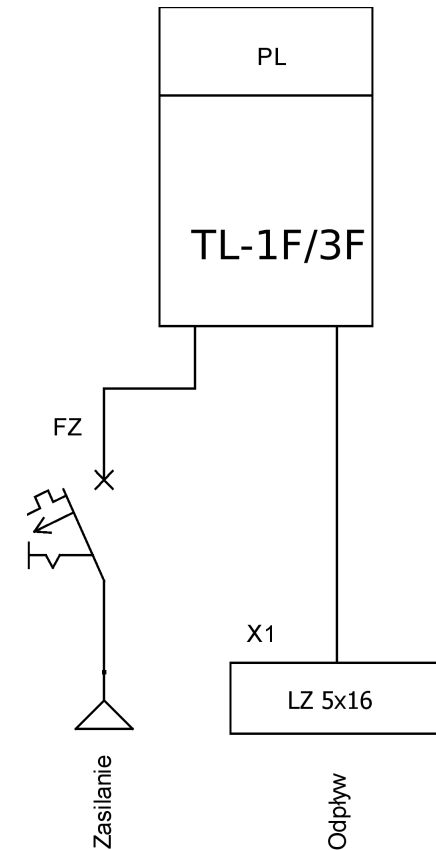
Schemat elektryczny
