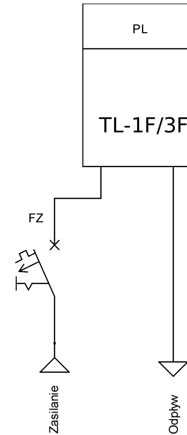
Schemat elektryczny
