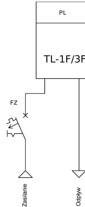
Schemat elektryczny
