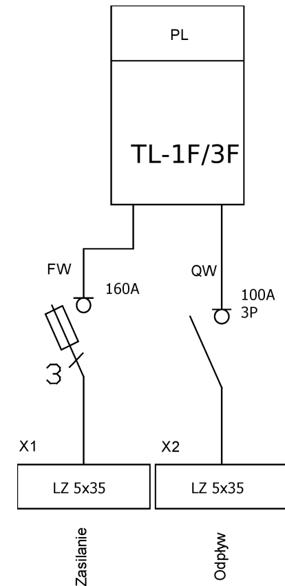
Schemat elektryczny
