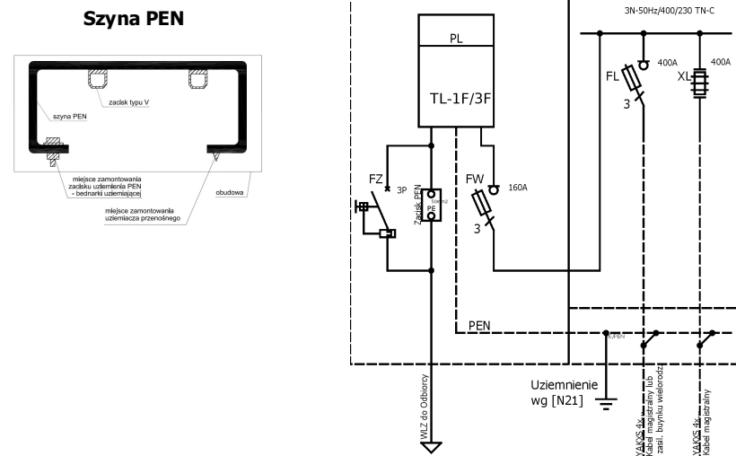
Schemat elektryczny
