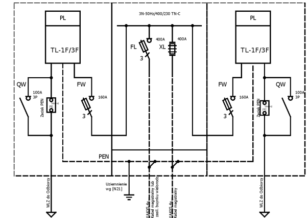
Schemat elektryczny
