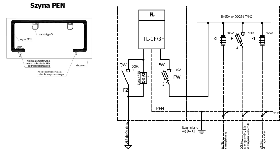
Schemat elektryczny
