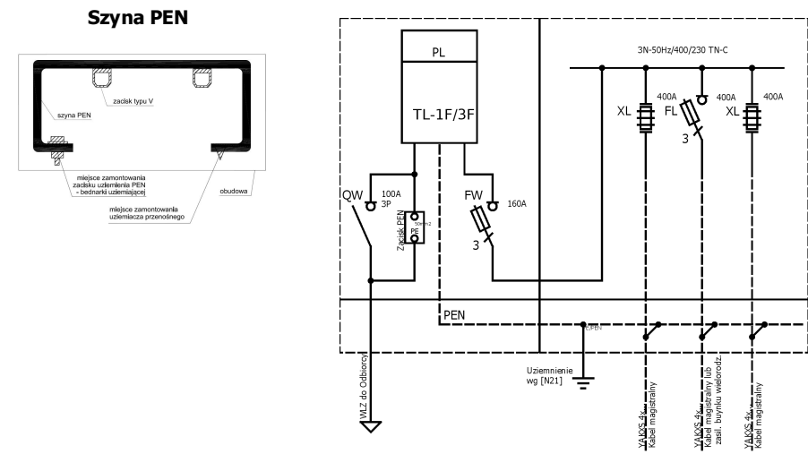
Schemat elektryczny
