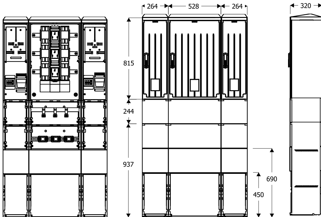
Widok złącza
