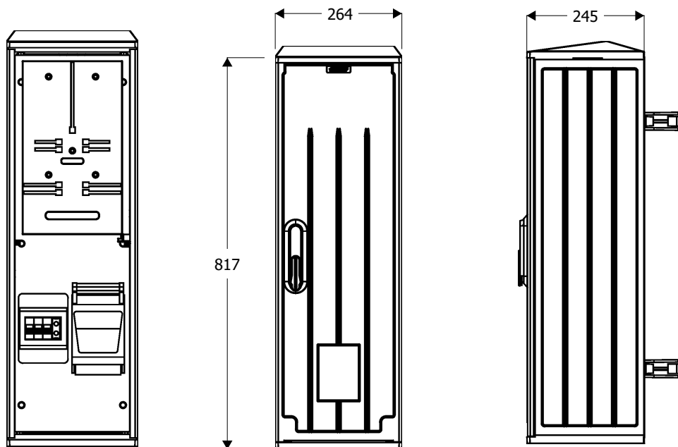
Widok złącza
