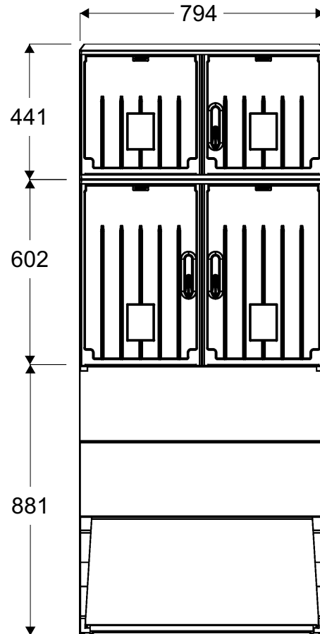
Widok złącza
