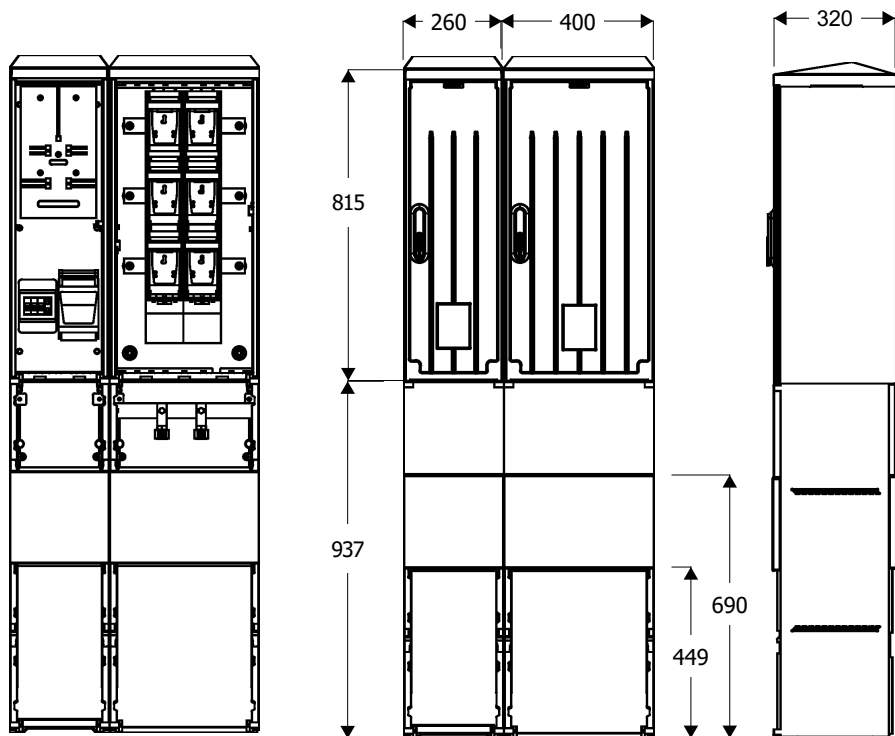
Widok złącza
