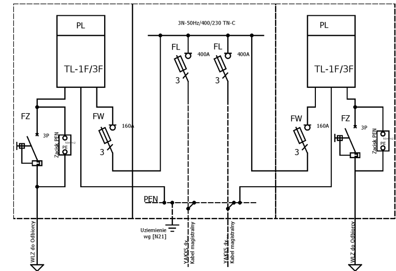
Schemat elektryczny
