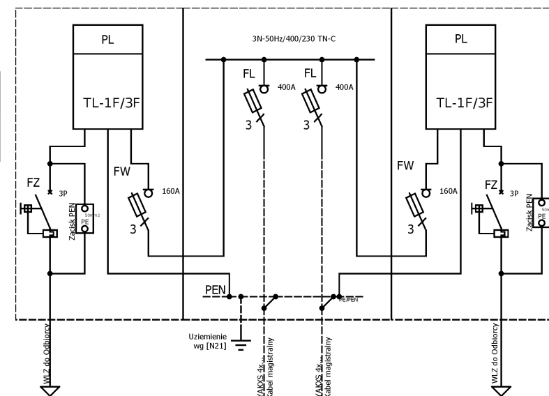
Schemat elektryczny
