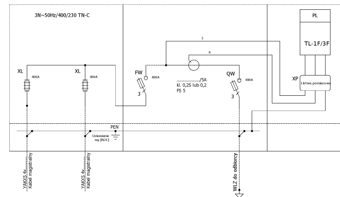
Schemat elektryczny
