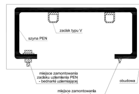
Szyna PEN
