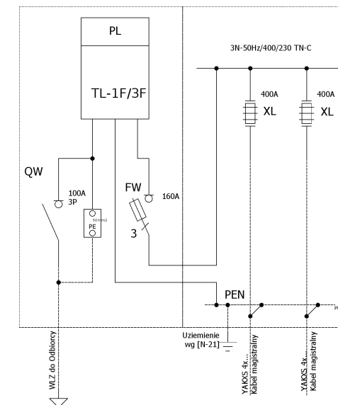
Schemat elektryczny
