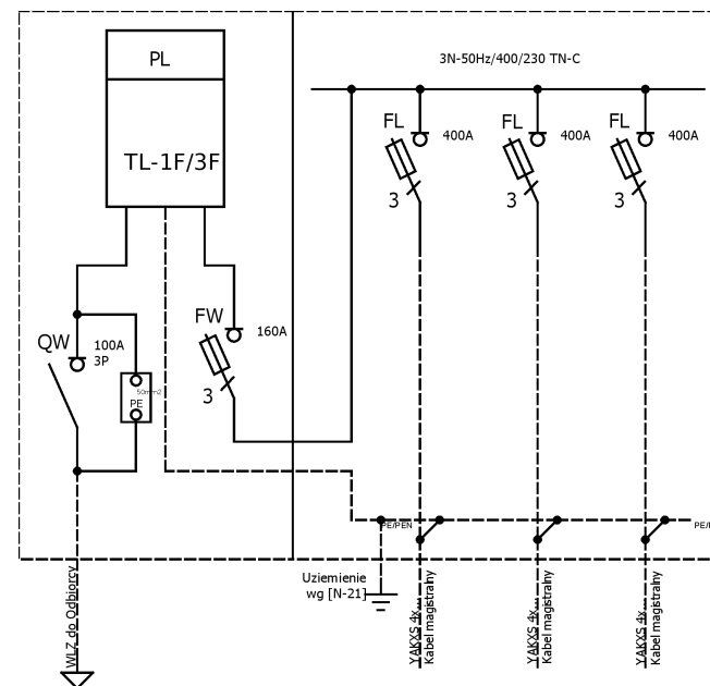
Schemat elektryczny
