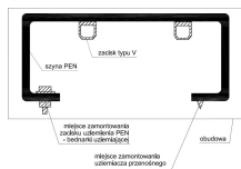
Szyna PEN
