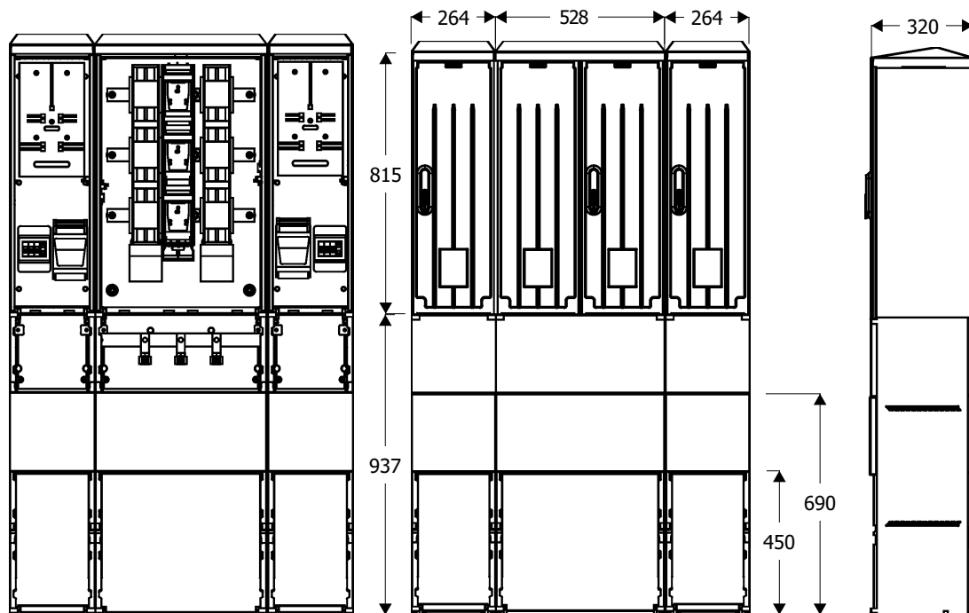
Widok złącza
