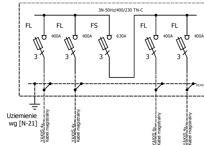
Schemat elektryczny
