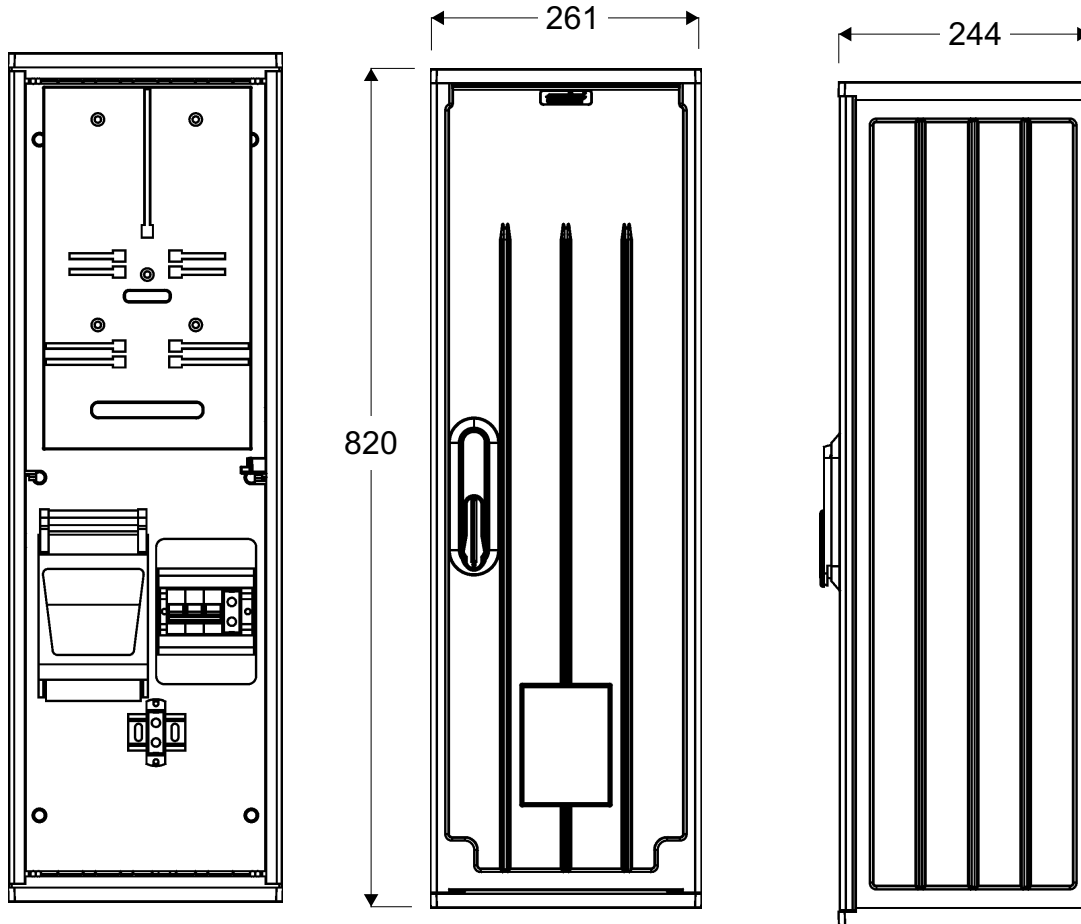
Widok złącza
