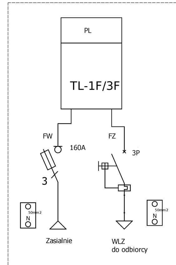
Schemat elektryczny
