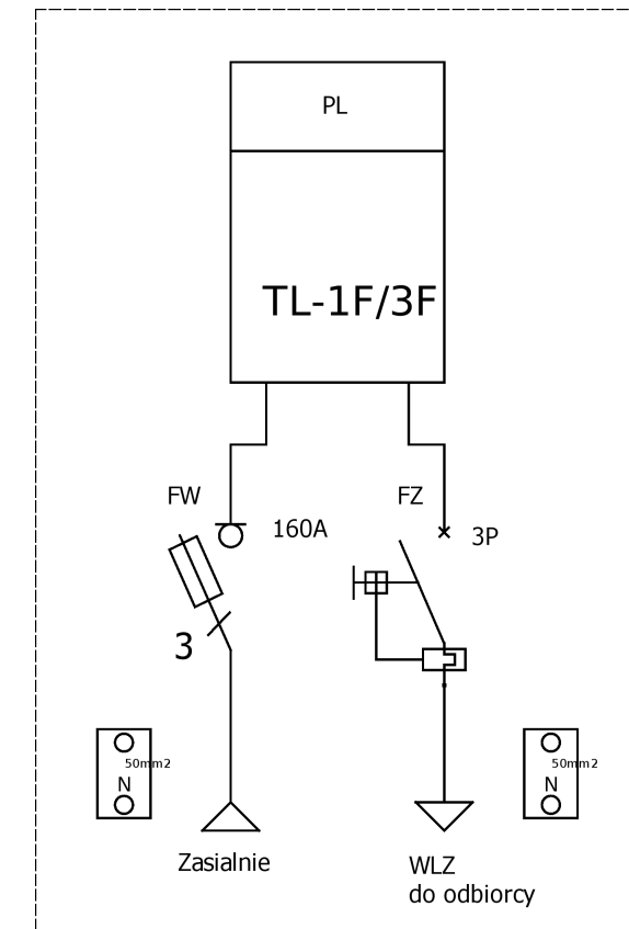
Schemat elektryczny
