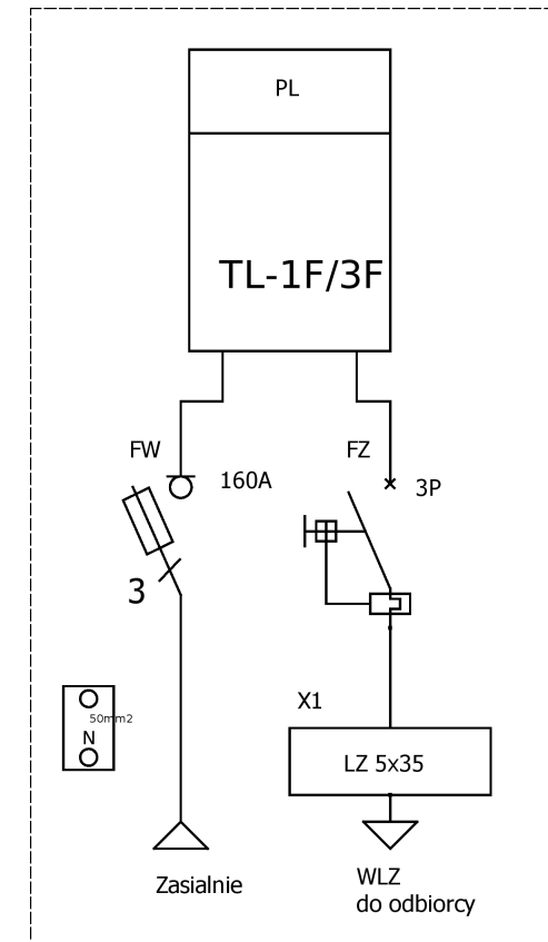
Schemat elektryczny
