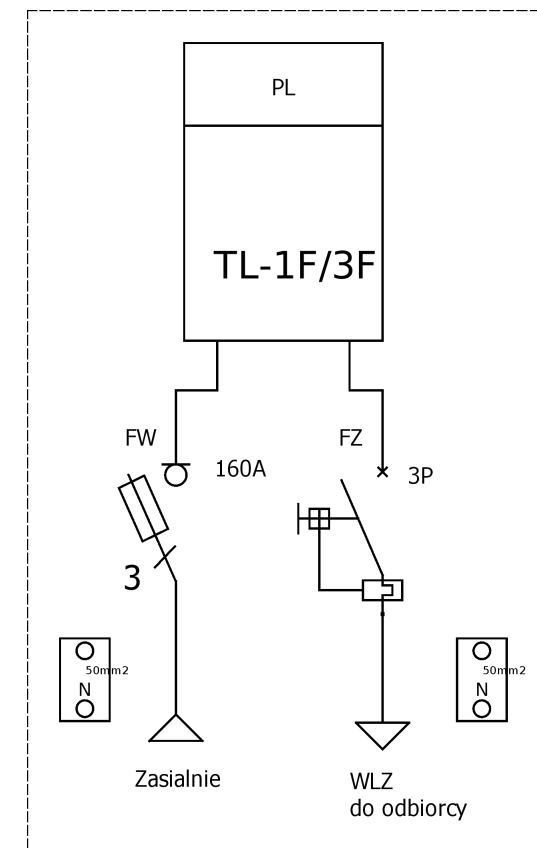
Schemat elektryczny
