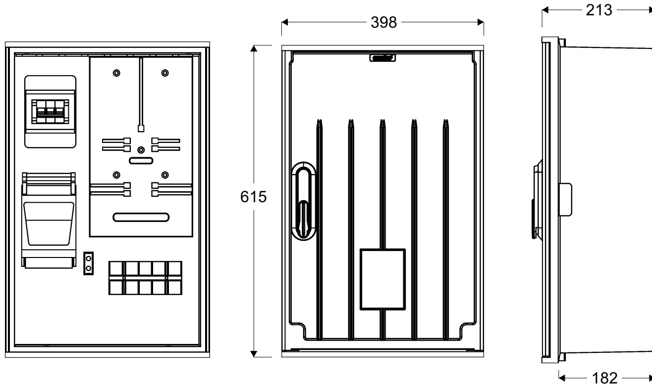
Widok złącza
