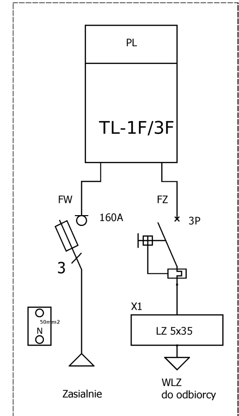
Schemat elektryczny
